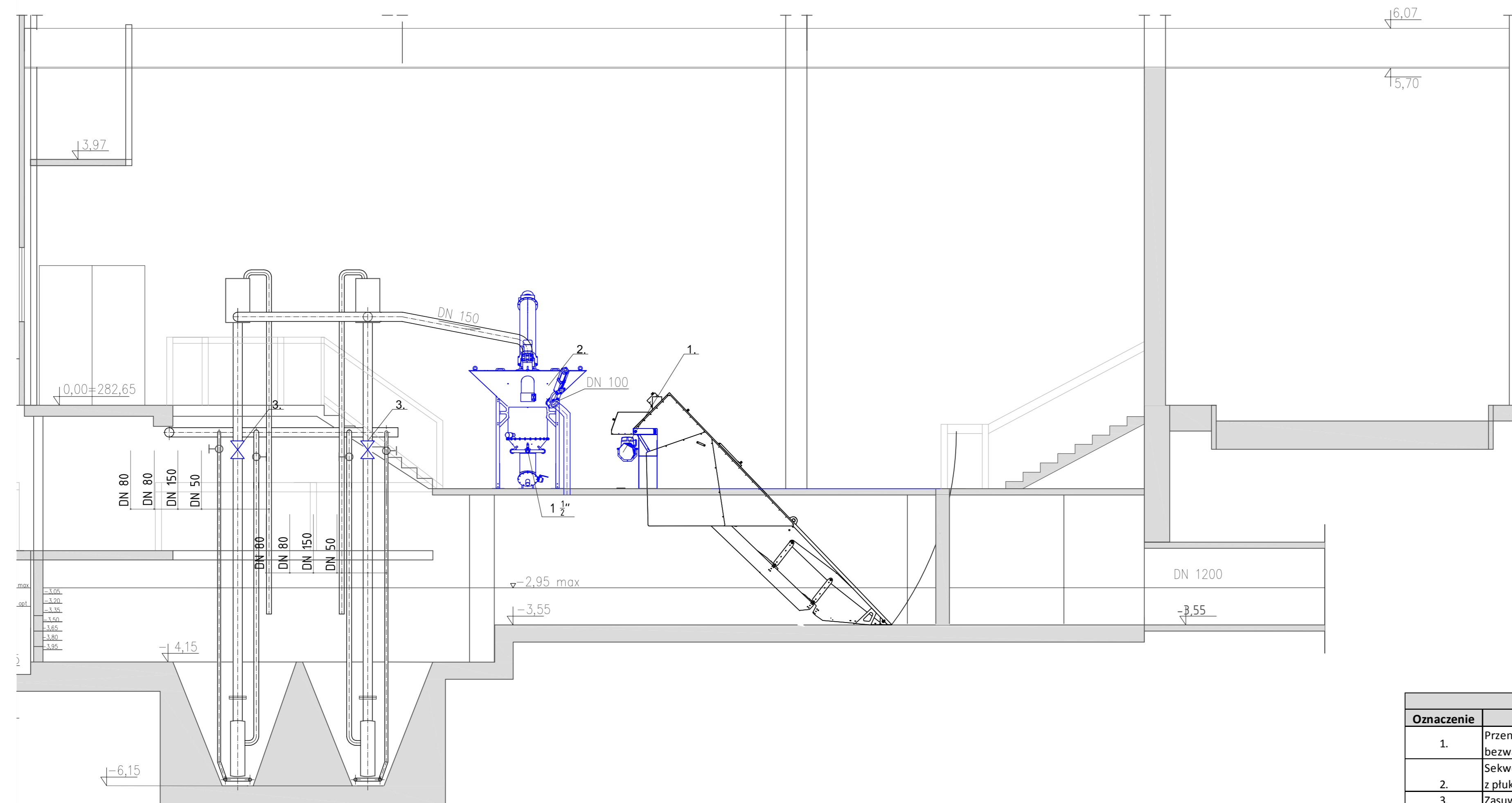
PRZEKRÓJ PODŁUŻNY 1-1
